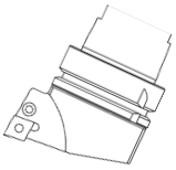
MCD' HSK-A63 F.26 PCLNR/L 065.12
