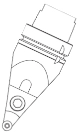
MCD' HSK-A63 F.77 SRDCN 130.12
