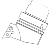
MCD' HSK-A63 F.26 PDJNR/L 070.15
